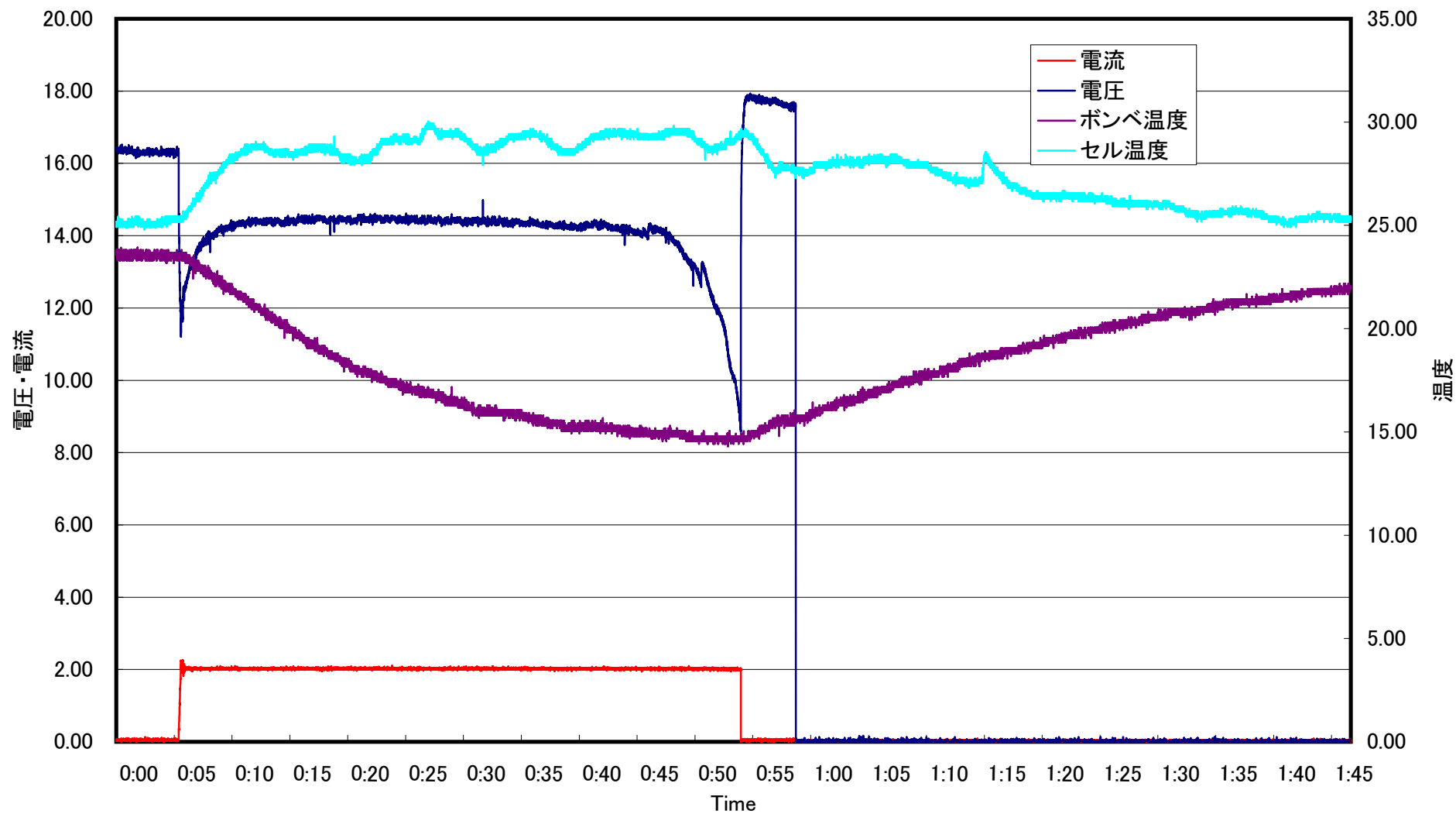
2A発電→停止特性
