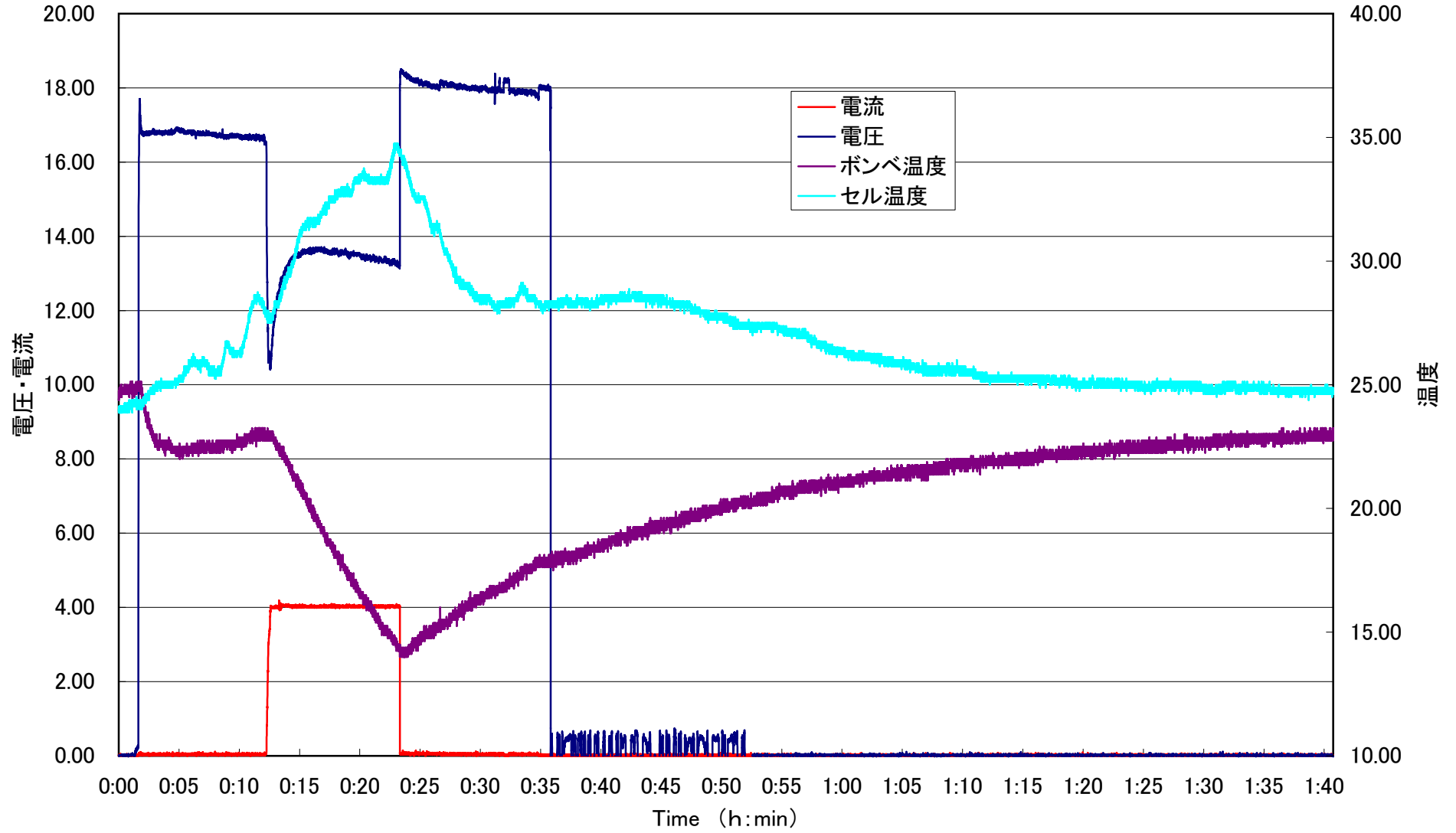
4A発電特性
