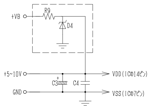
電源部
