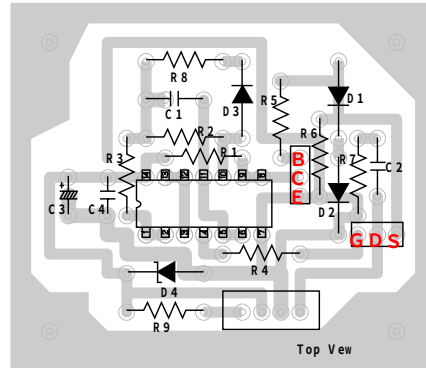
基板部品面配置図
