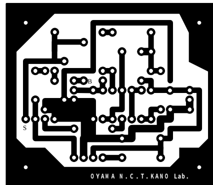
基板配線面パターン図
